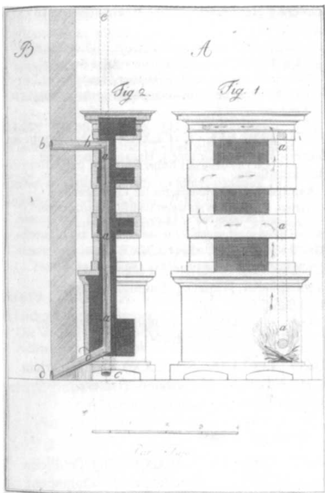
Abb. 3: Circulierterröhren-Heizung
